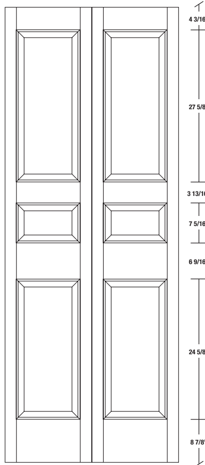
2035P / 2935P
